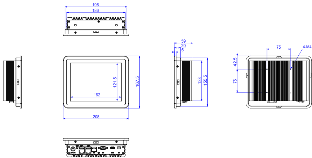
产品外形尺寸图
